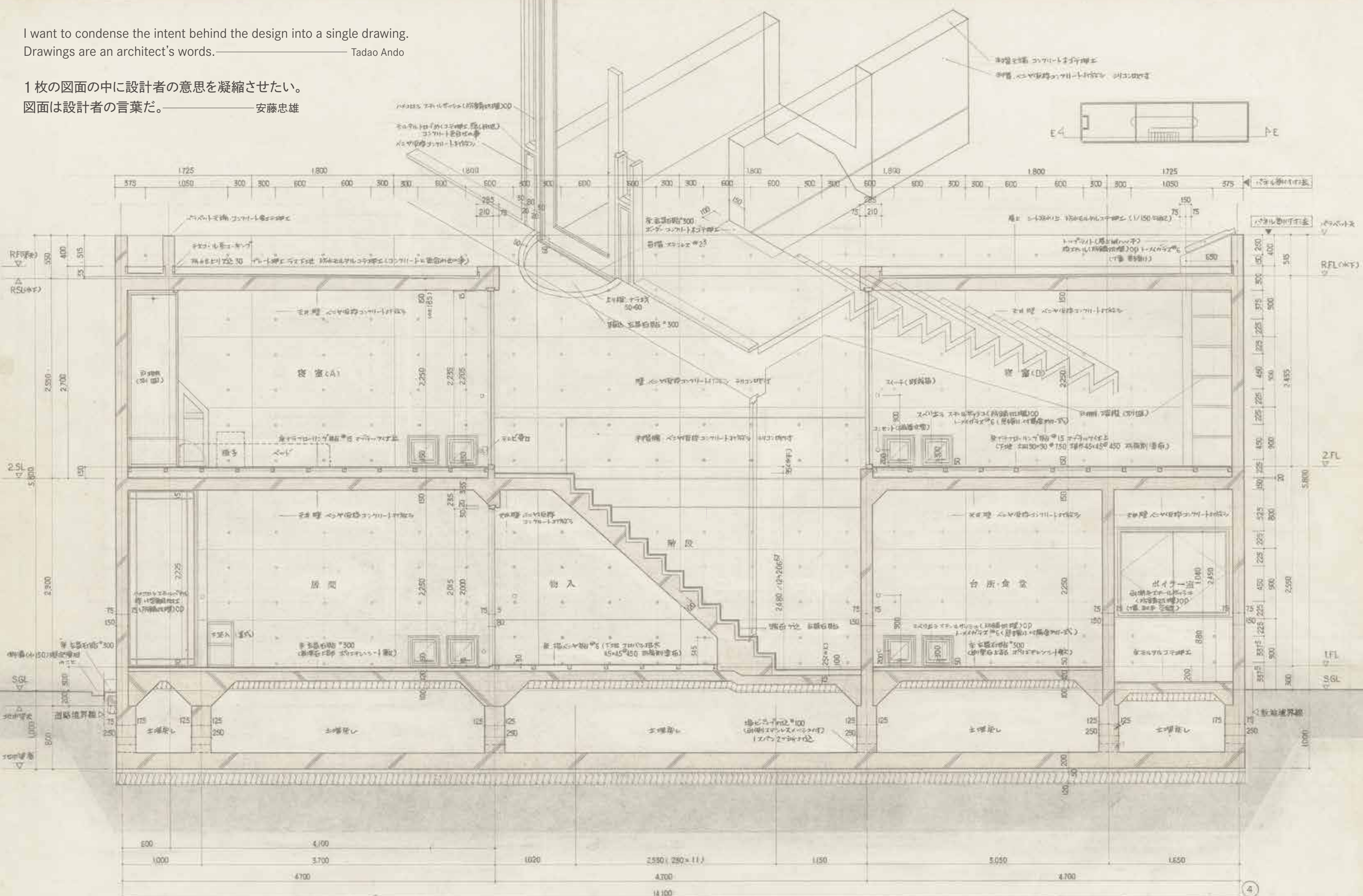
断面詳細図 E-E' 1/30
