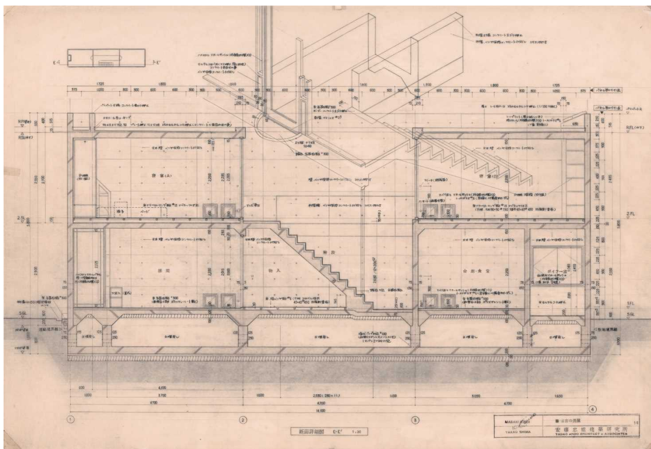
住吉の長屋 断面詳細図
