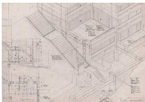
六甲の集合住宅Ⅰ アイソメ図
