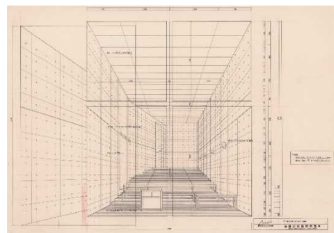
光の教会 透視図
