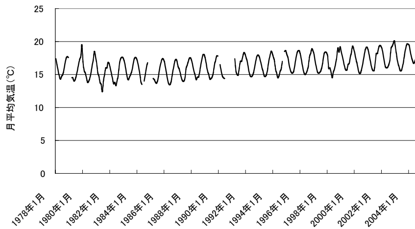
図 2. 高松塚古墳石室内 (下) 気温の変動
