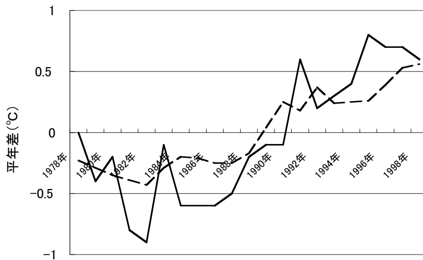
図 6. 高松塚古墳とラスコー洞窟における平年差の推移
