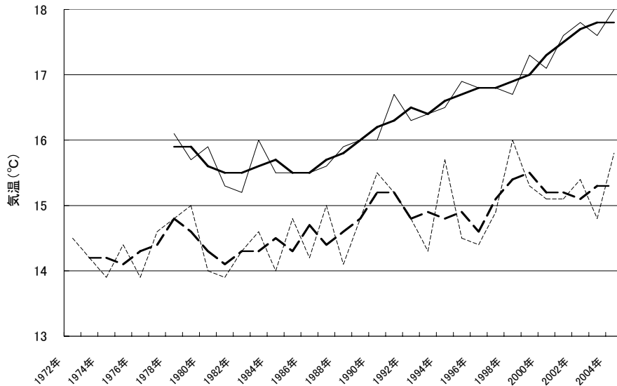
図 3. 高松塚古墳石室内年平均気温の経年変化
