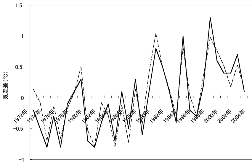
図 5. 気温の平年差の経年変化（奈良、日本）
