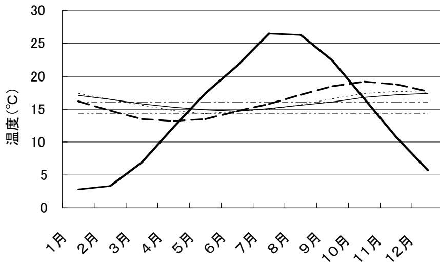
図 4. 橿原における気温と地温の変化
