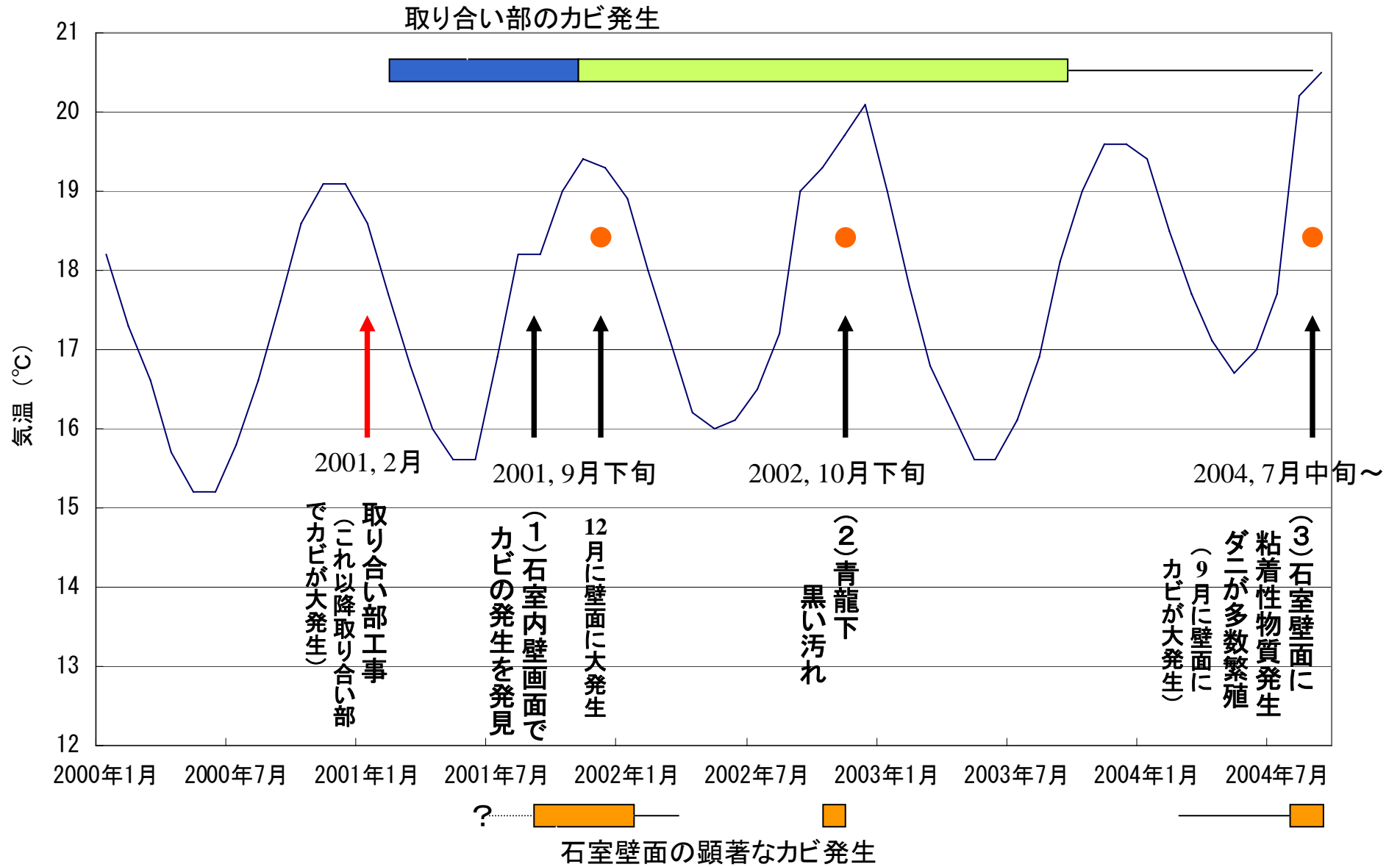
高松塚古墳石室内温度変化（2000-04年）
