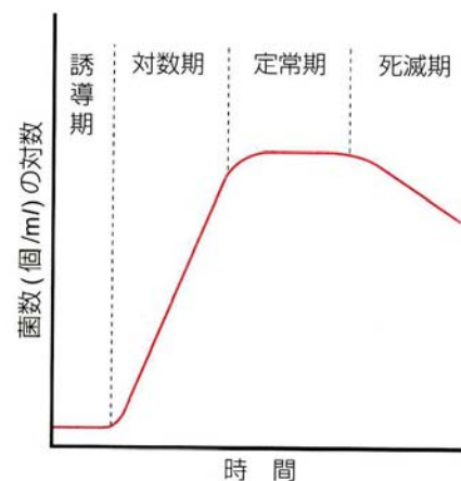
図 6.6 ●微生物の成長曲線
