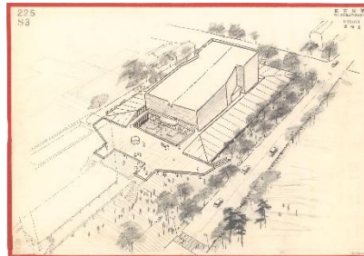
菊竹清訓 | 萩市民館 透視図 | 1967 | 国立近現 代建築資料館所蔵 KIKUTAKE Kiyonori | Hagi Civic Center, Perspective Drawing | Courtesy of National Archives of Modern Architecture
