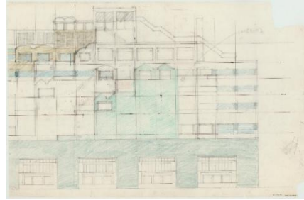
原広司+アトリエ・ファイ建築研究所 | ヤマト トインターナショナル 立面スケッチ | 国立近 現代建築資料館所蔵 HARA Hiroshi + Atelier Phi | Yamato International, Sketch of Elevation | Courtesy of National Archives of Modern Architecture
