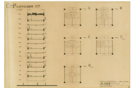
大高正人 | 広島市基町団地・広島県長寿園団 地 長寿園団地住居単位計画図 | 1969 | 国立近 現代建築資料館所蔵 OTAKA Masato | Motomachi Apartments, Chojuen Apartments, Chojuen Apartments Unit Plan | Courtesy of National Archives of Modern Architecture
