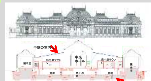
《京都国立博物館耐震改修イメージ》
