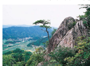
大滝山の険しさを象徴するチャートの巨岩
