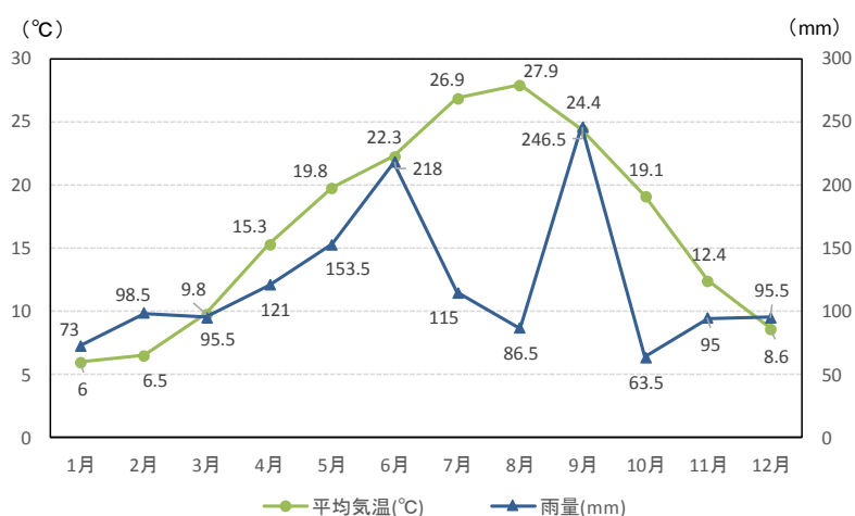
平均気温と雨量（平成 28 年（2016 年））
