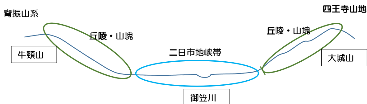
図 37 : 地形特性図
