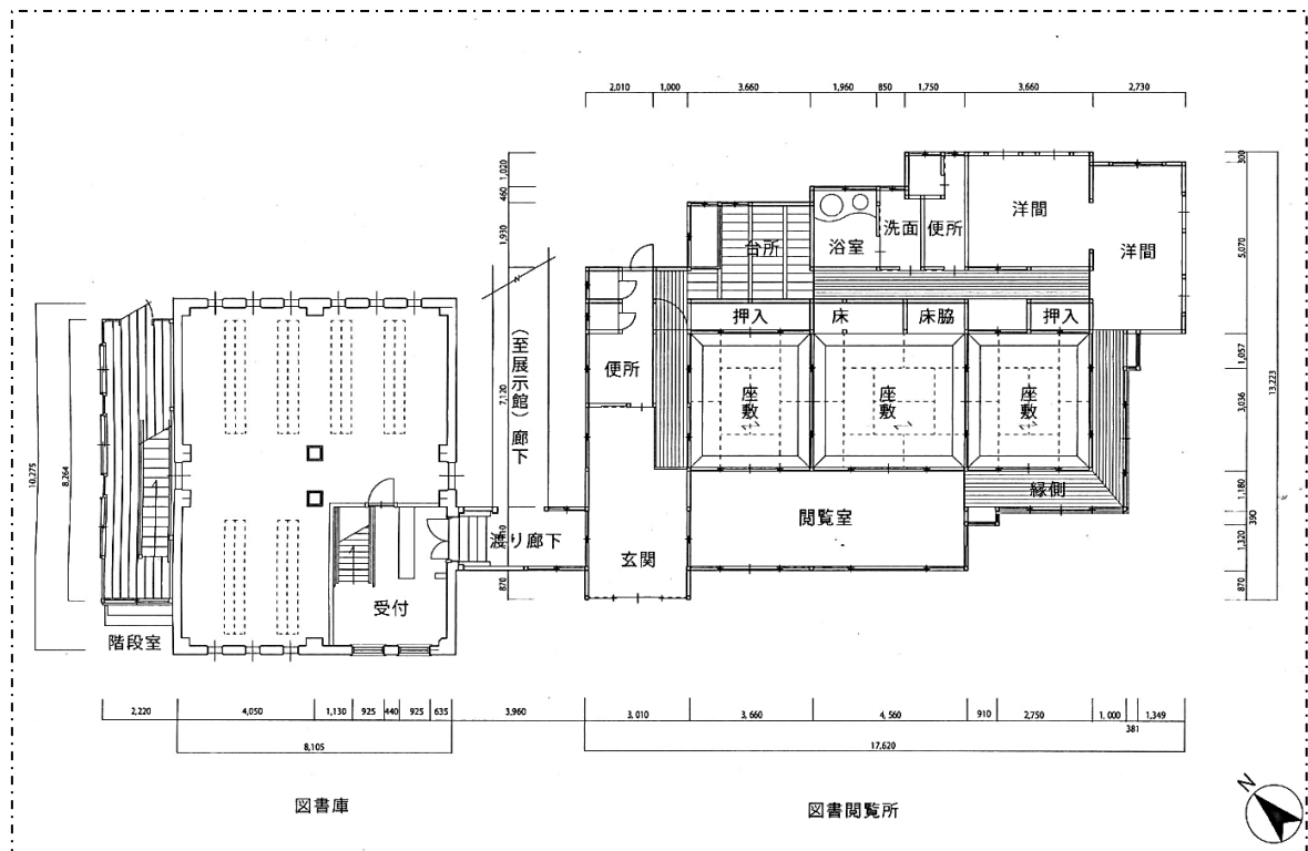
図 1-2 平面図の作成例
